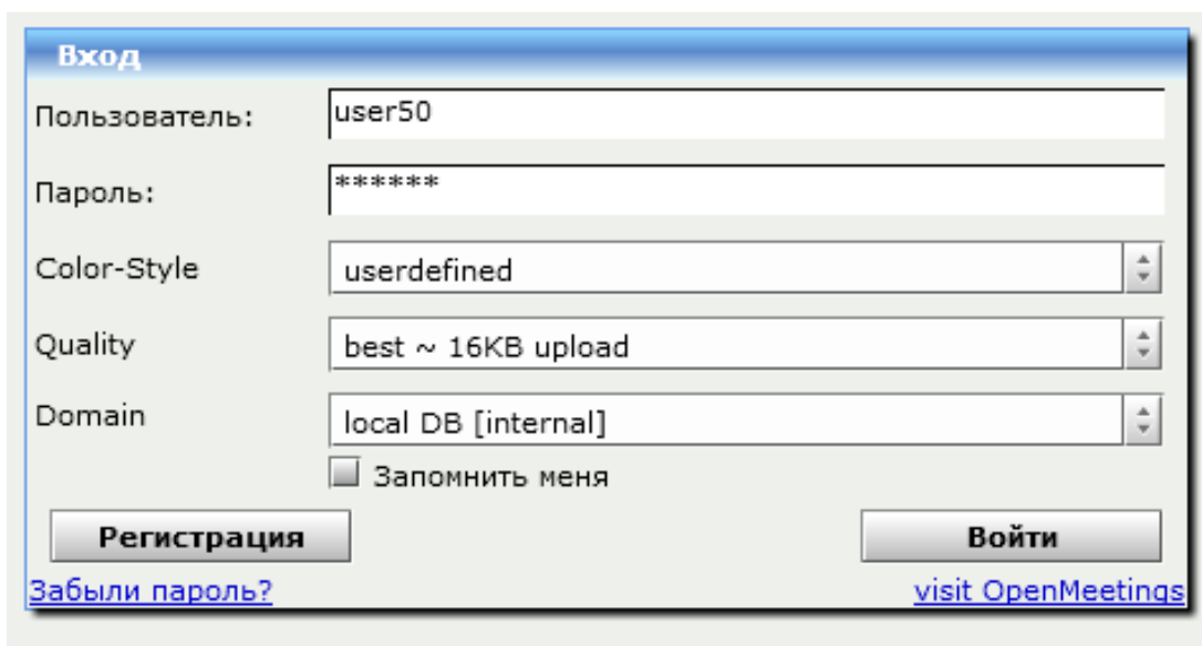
Рисунок 2 – Окно авторизации
